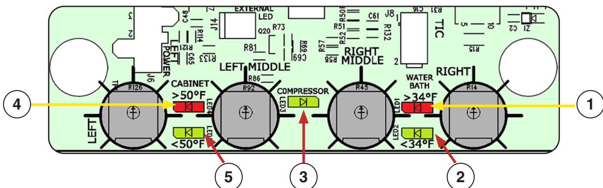
Indicadores LED de la placa de control
