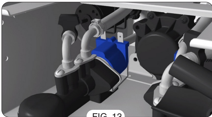
FIG. 13 Válvula dosificadora izquierda con accesorios asegurados.
