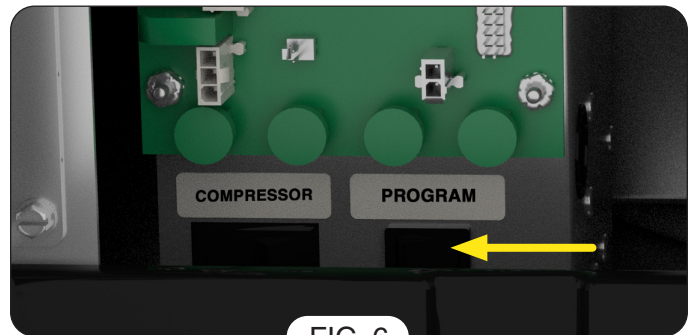
FIG. 6 Interruptor de programa
